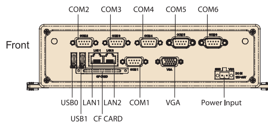
ARK-3360F 外置I/O视图
