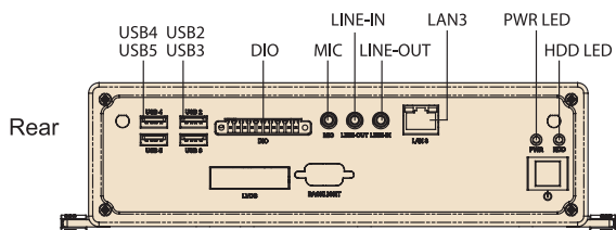
ARK-3360F 外置I/O视图
